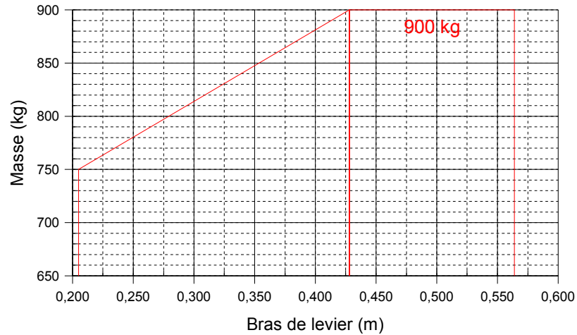
Enveloppe de centrage
